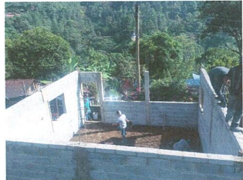
Foto 4: Instalación de piso de concreto
